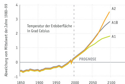
A1, A1B, A2 = verschiedene Szenarien Quelle: Quelle IPCC
